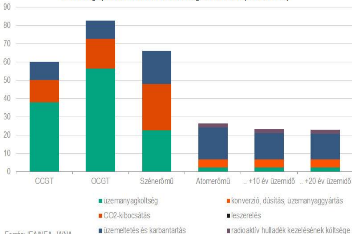
Már megépült erőművek önköltségszerkezete (USD/MWh)
