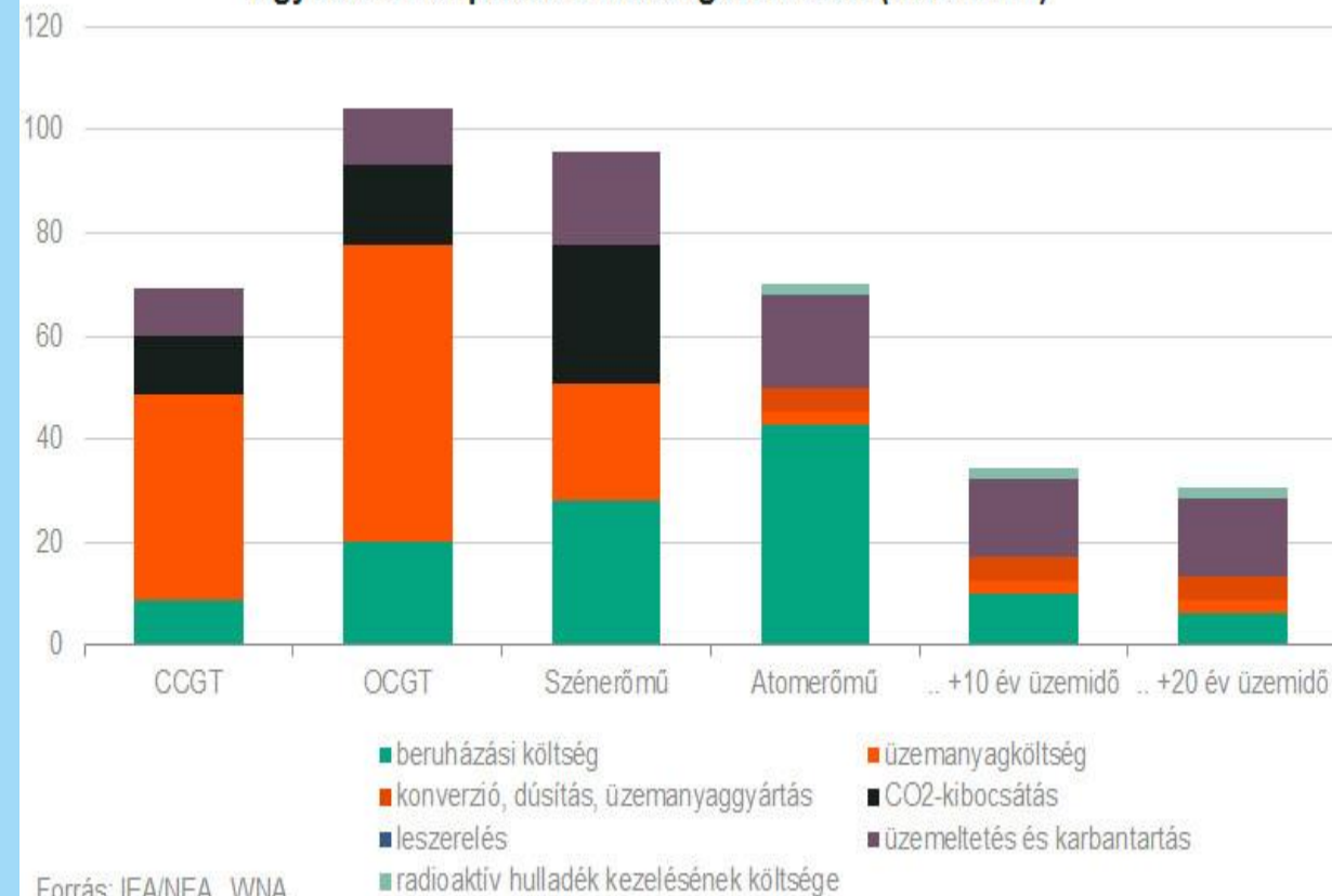
Egyes erőműtípusok önköltségszerkezete (USD/MWh)
